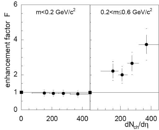
(b) CERES
